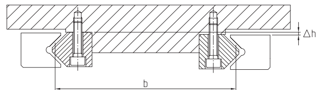
Bild 22. Höhenversatz bei geschlossener Anordnung
