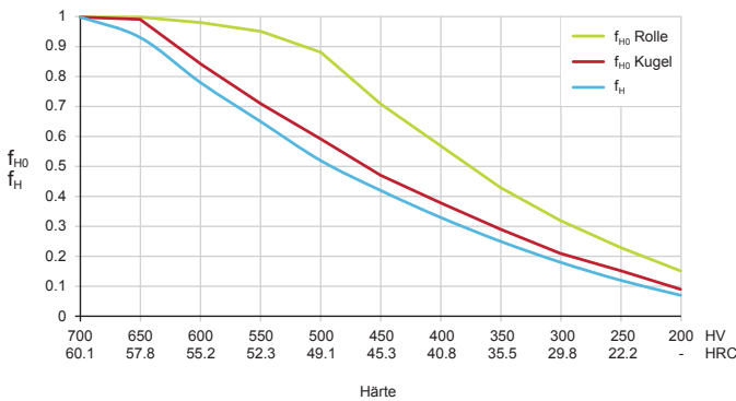
Bild 10. Härtefaktoren
