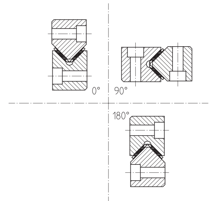
Fig. 21. Positions de montage
