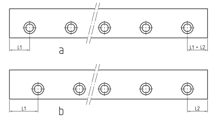
Fig. 6. Positions de perçage symétrique (a) et asymétrique (b) d'une rangée de trous
