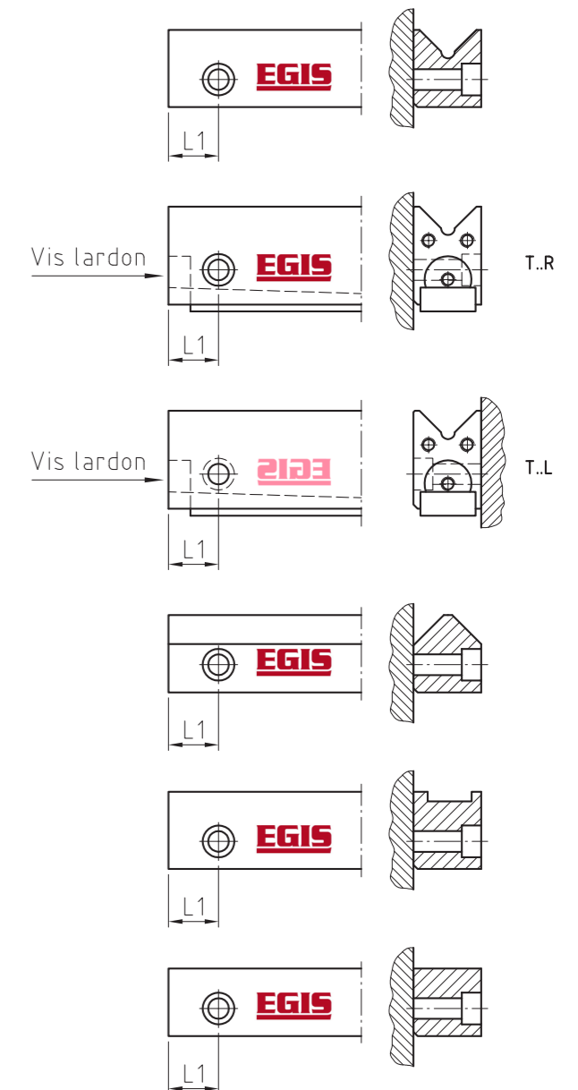
Fig. 7. Position de la distance entre le premier trou de fixation et le début du rail L1 selon le type de rail.
