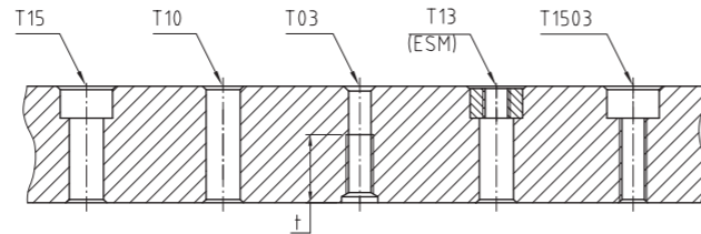
Fig. 4. Types de trous de fixation
