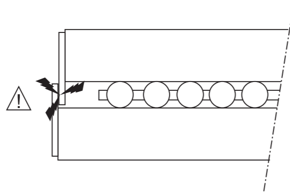
Fig. 8. Montage erroné de plaquettes d'arrêt ou de racleurs
