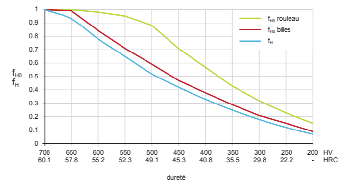
Fig. 10. Facteurs de dureté
