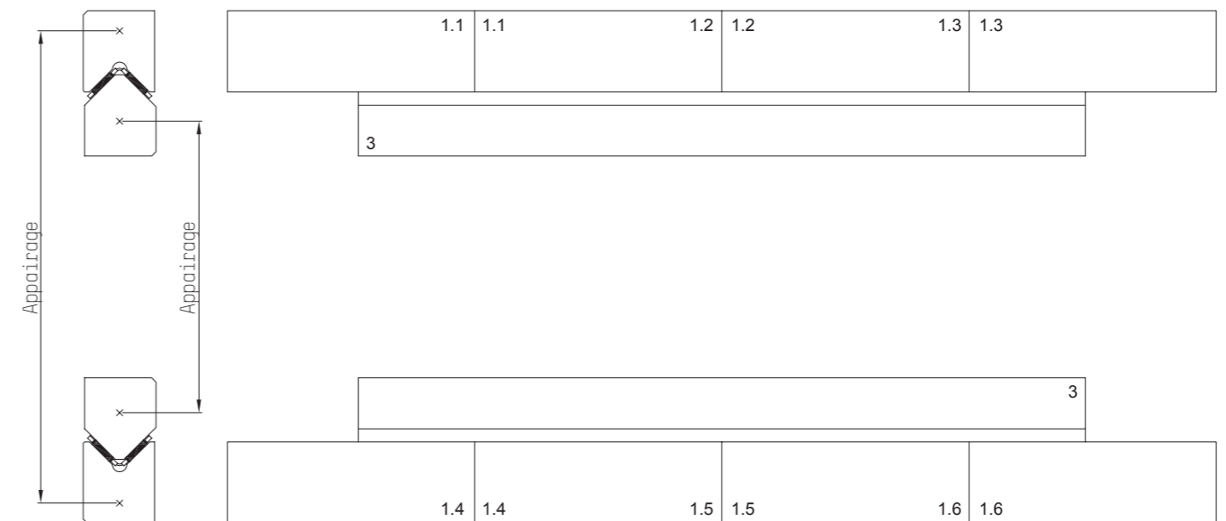
Fig. 24. Numérotation sur rails de guidage en un et plusieurs éléments
