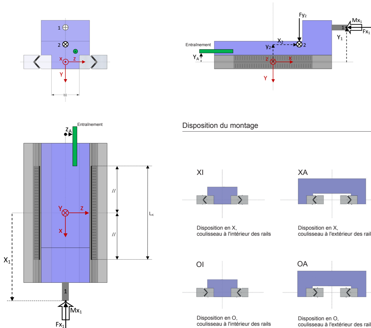
Fig. 15. Géométrie et données de la charge
