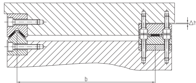
Fig. 23. Compensation de la différence de hauteur à l'aide d'une cale dans le cas d'une construction ouverte.
